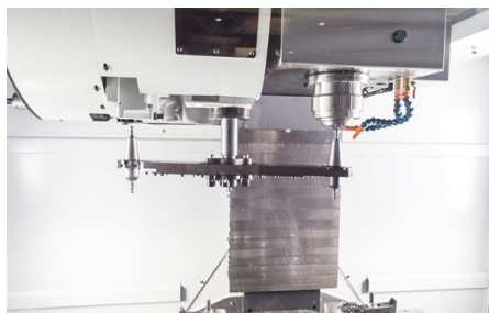
Cambiautensili con doppio braccio e mandrino
