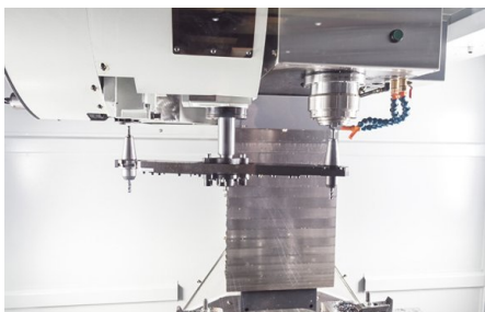
Cambiautensili con pinza a doppio braccio e 24 postazioni
