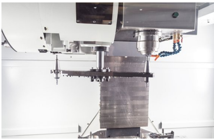
Il cambiautensili con pinza a doppio braccio e 24 postazioni consente brevi tempi di cambio
